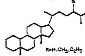
XXVI. dfastranes
