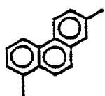
XI. pimaratriene
