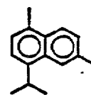
III. cadalene
