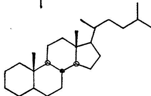
Xvi. Norcholestane
