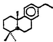
XII. 17-norddehydroabietane
