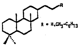
XVI. extended diterpanes
