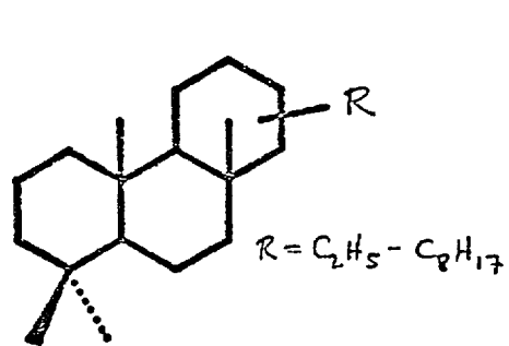
I. Extended diterpanes
