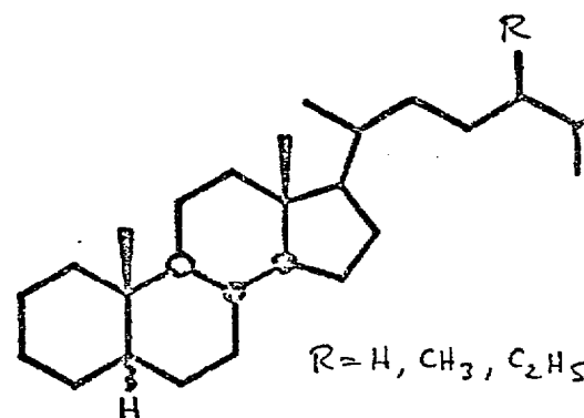
X. 8\beta, 14\beta(H) -Steranes
