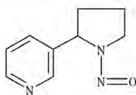
N' -nitrosoanatabine
