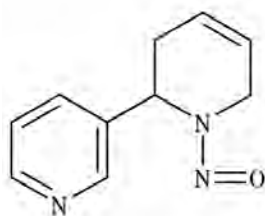
N' -nitrosoanatabine
