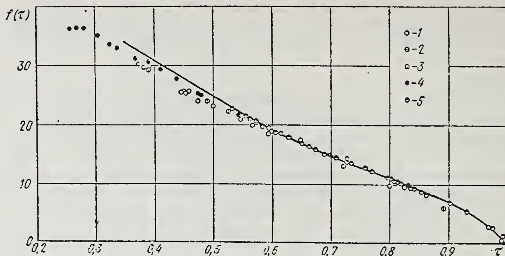
Figure 18. Values of functions f(\tau) in expression (64) according to: 1 -- N. S. Rudenko [29]; 2 -- N. S. Rudenko [30]; 3 -- S. F. Gerf and G. I. Galkov [31, 32] (ethylene); 4 -- S. F. Gerf and G. I. Galkov [31, 33]; 5 -- I. A. Neduzhiy and Yu. I. Khmara [34].
