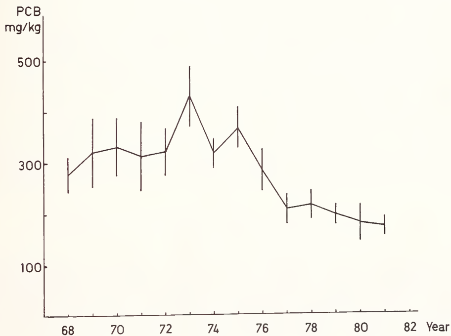
Figure 3. Mean levels of PCB and 95% confidence interval in eggs of Guillemot Uria aalgae collected at Stora Karlsö in the Baltic Sea proper during 1968-1981. From M. Olsson & L. Reutergårdh, Kommitten för Bottniska Viken. Årsrapport nr 10 (1982)
