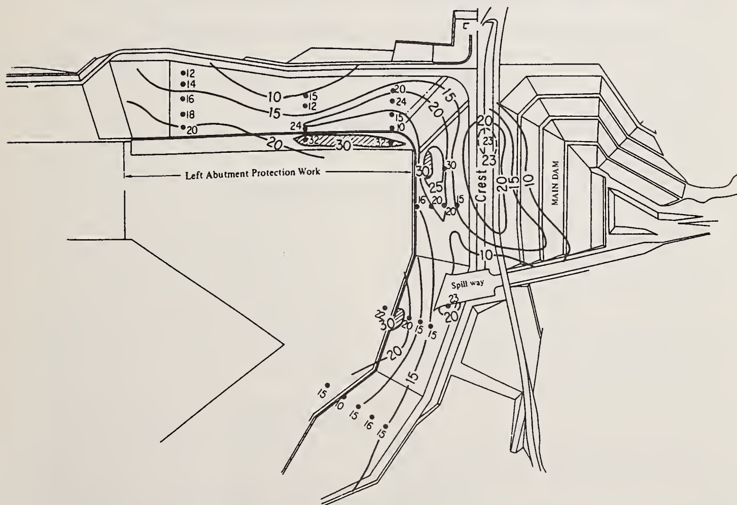
図-15 長柄ダムにおける沈下
