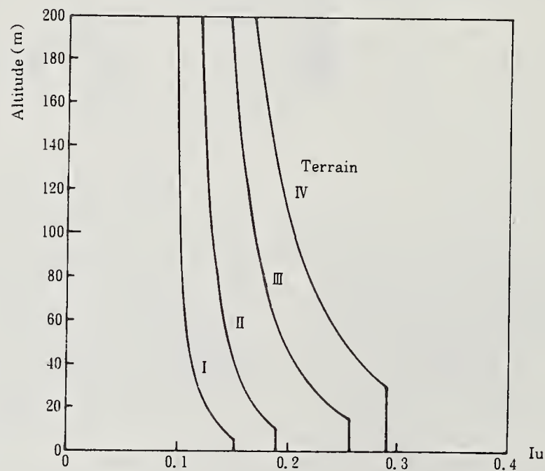
Fig. 4 Trubulence intentity
