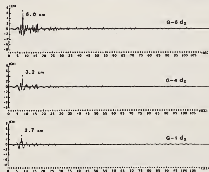
(b) Displacement
