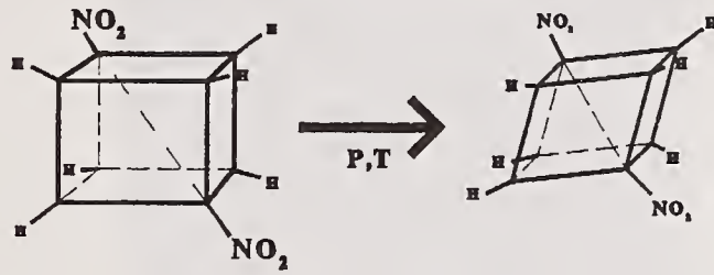
1,4 DINITROCUBANE
