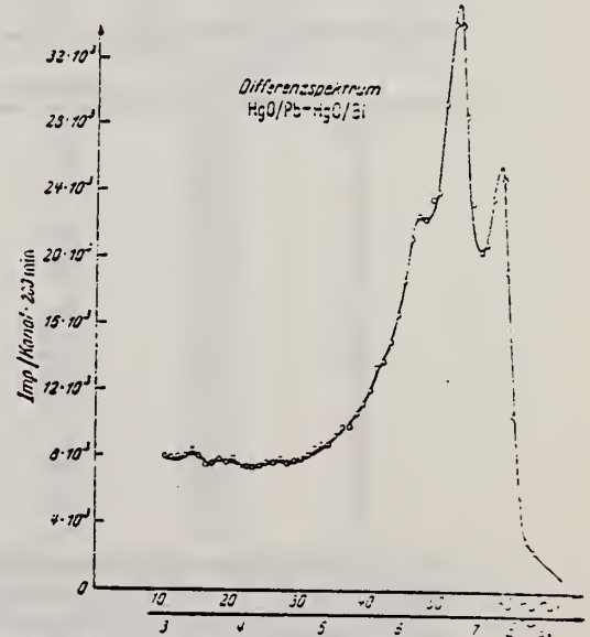
Fig. 2. Spektrum der eigentlichen Resonanzstreuung (Differenz der Spektren von Fig. 1)
