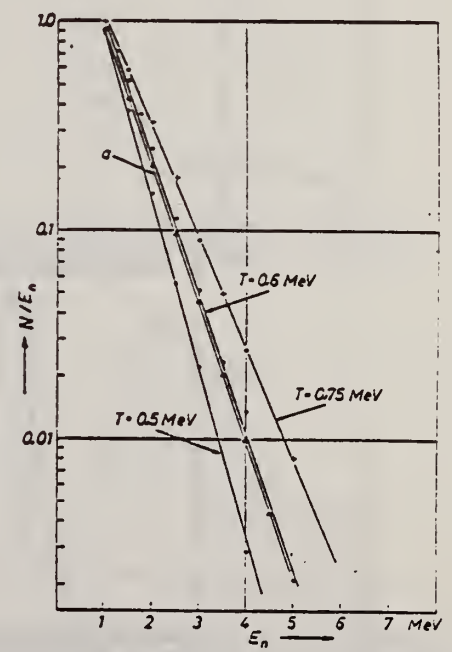
Abb. 11. \ln N/E_n als Funktion der Neutronenenergie E_n .
