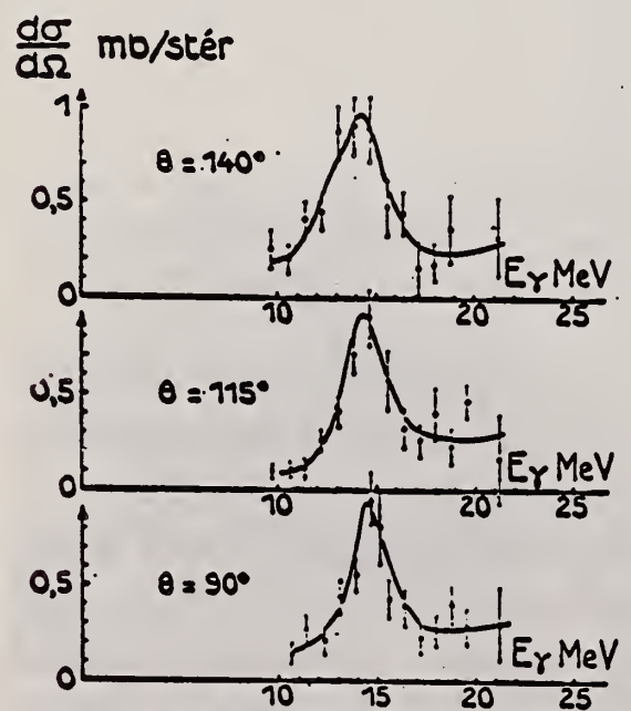
FIG. 6. — Distribution angulaire des photons diffusés élastiquement sur Bi.
