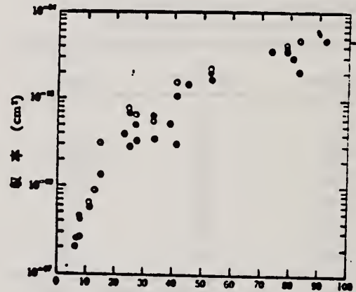
●: 実験値, ⊕: Johnsら, ⊙: Nathansら, ○: Montalbettiら 図4 ( \gamma, n )反応の収率の比較
