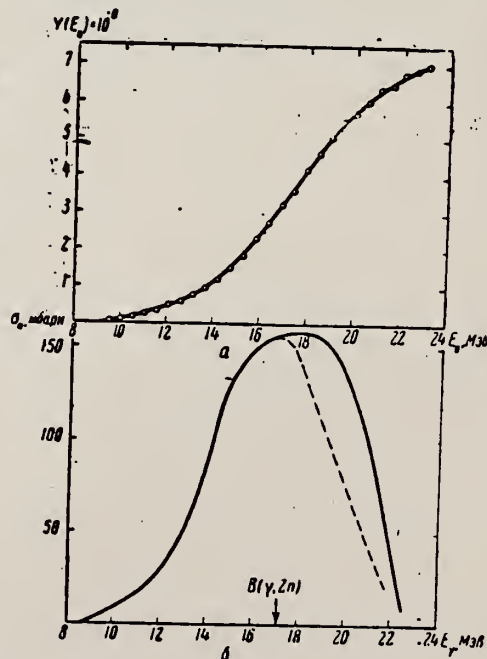
Рис. 6. а — Выход фотонейтронов для Nb; б — \sigma_n(E_\gamma) и \sigma(\gamma) для Nb
