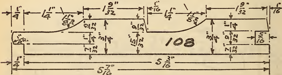
FIG. 29.—Drop siding
