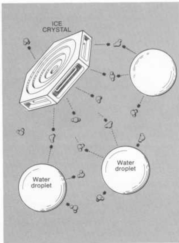
VAPOR
