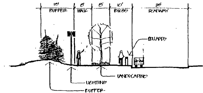
BELLE RUE ENTRY SEGMENT P
