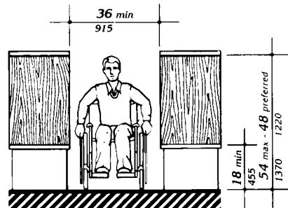
Fig. 55 Card Catalog
