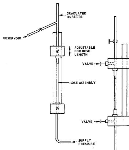
FIG.1.EXPANSIONTEST APPARATUS
